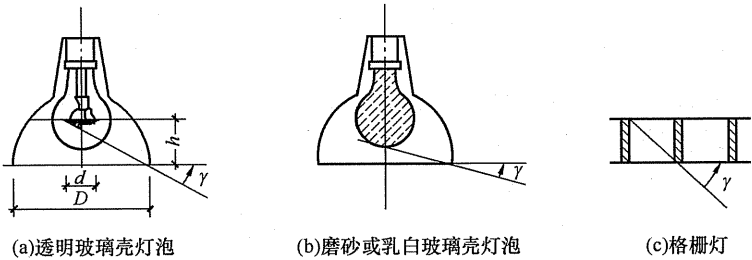
图 2 遮光角示意
